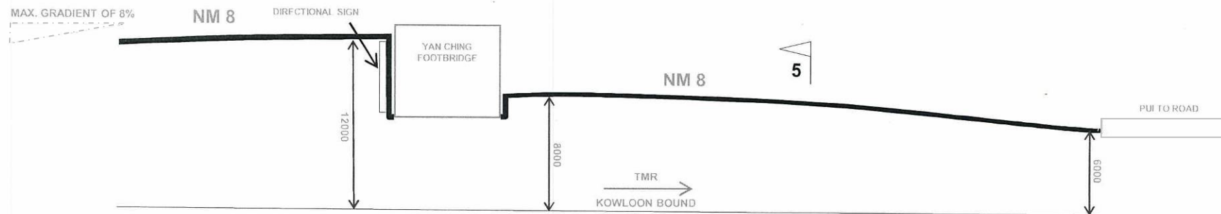
LONGITUDINAL SECTION ALONG TMR KOWLOON BOUND NM8 (N.T.S.)
